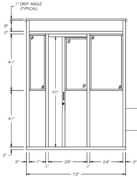
E1 LEFT ELEVATION SCALE \frac{1}{2}'' = 1' - 0''
