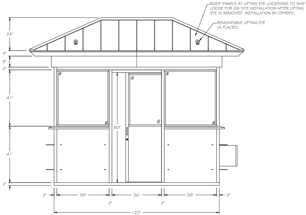
E1 LEFT ELEVATION SCALE \frac{1}{2}'' = 1' - 0''
