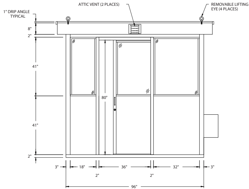
E1 LEFT ELEVATION SCALE \frac{1}{2}'' = 1' - 0''
